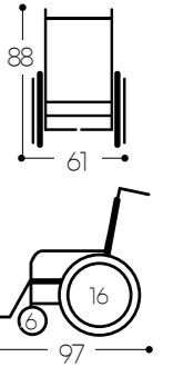
수동휠체어 MIRAGE2(16D) M18030043004
