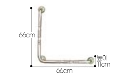
안전손잡이 YGW-L F18030045108
