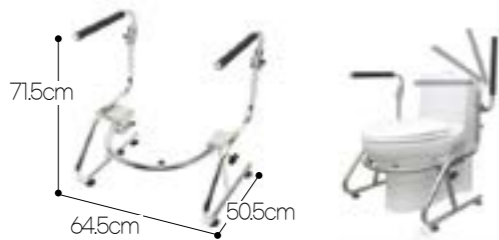
안전손잡이 MSH-502 F18030034104
