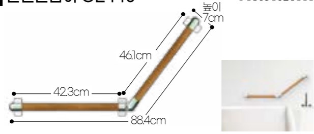
안전손잡이 CE440 F18031026111
