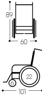
수동휠체어 MIRAGE7(22D)-B M18030043014
