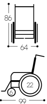
수동휠체어 MIRAGE(22D) M18030043005
