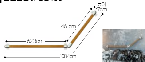
안전손잡이 CE460 F18031026108
