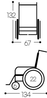
수동휠체어 HAL-48(22D) M18030043002
