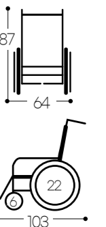
수동휠체어 DS-921BB M18031074101
