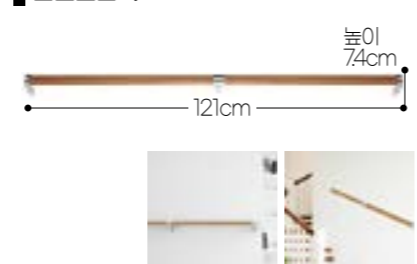
안전손잡이 CC1200 F18031026103
