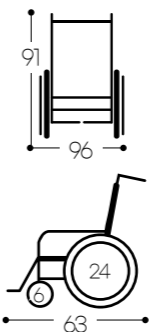
수동휠체어 BH-H01 M18031113602
