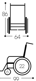
수동휠체어 MIRAGE(22D)-P M18030043103
