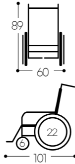
수동휠체어 MIRAGE7(22D) M18030043001
